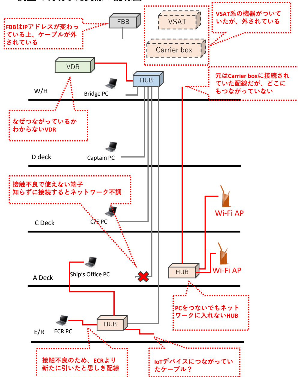
調査で判明した実際の配線図
